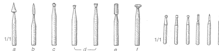
Ryc. 2.5. Wiertła diamentowe: a – stożek, b – płomień, c – kulka, d – odwrócony stożek, e – wałek, f – krążek.
