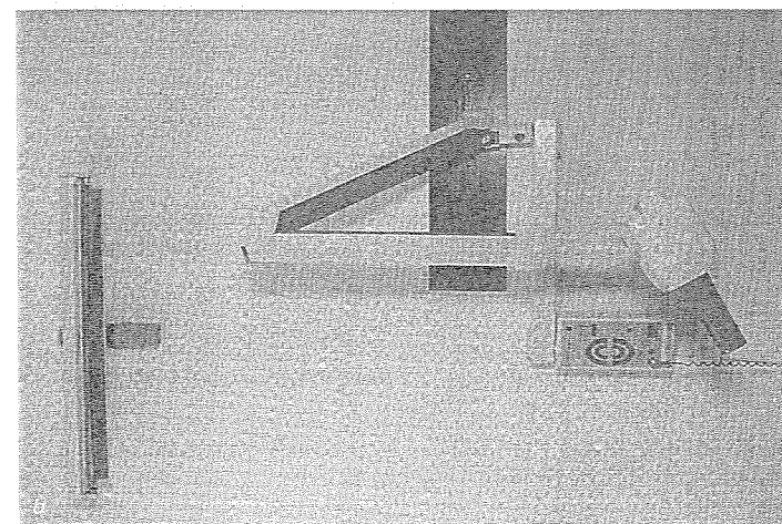
Ryc. 8.2. Typy aparatów rentgenowskich, stosowanych w diagnostyce stomatologicznej: a – aparat do zdjęć pantomograficznych – Ortopantomograph-OP 100; b – aparat do zdjęć zębowych – Trophy CCX Digital (pracownia rentgenowska Elcomed).
