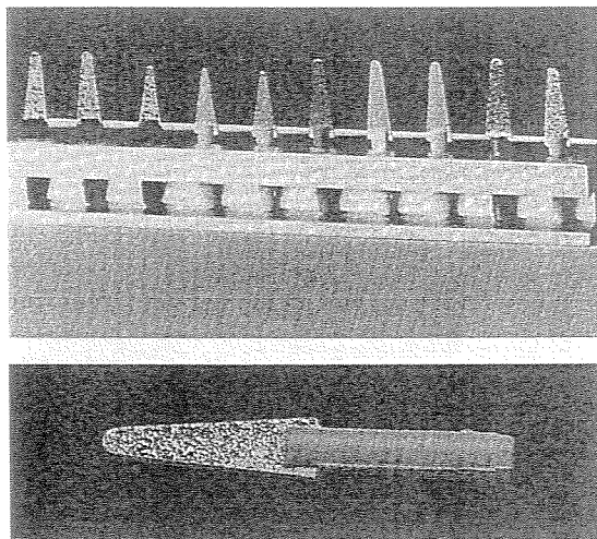
Ryc. 16.34. Zestaw pilniczków diamentowych i wolframowych do kątnicy Profin.
