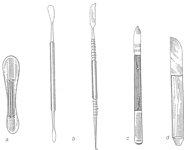
Ryc. 2.46. Łopatki i nożyki: a – łopatką do przygotowania masy wyciskowej, b – łopatką do wosku, c – nożyk do wosku, d – nóż do gipsu.
