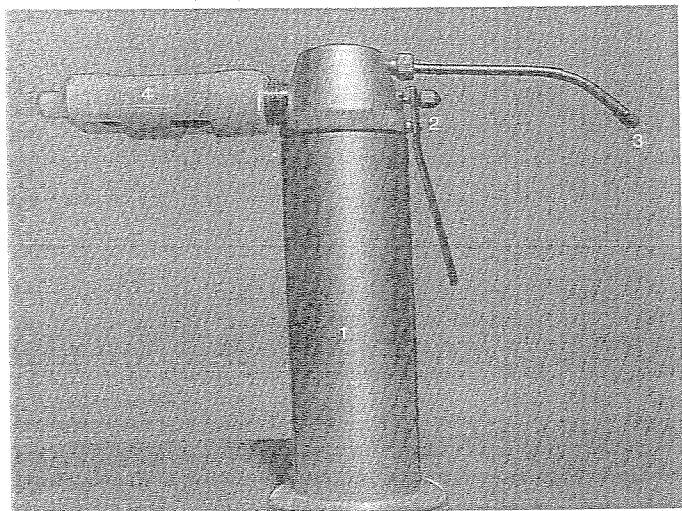
Ryc. 9.2. Atomizer: 1 – pojemnik na lek, 2 – przycisk otwierający zawór wylotowy, 3 – dysza wylotowa, 4 – pojemnik na nabój do autosyfonu.
