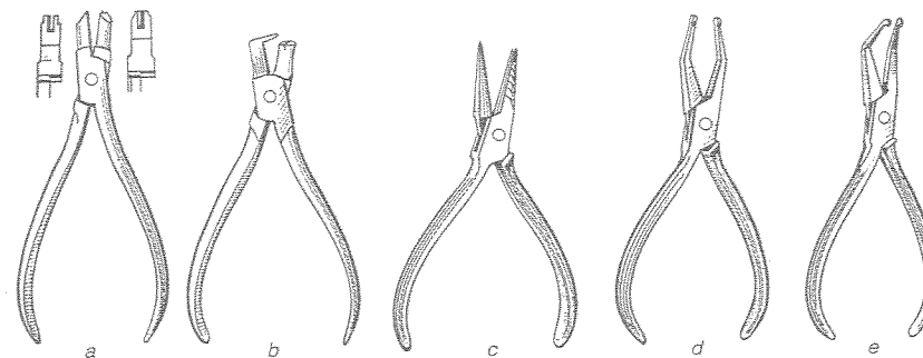
Ryc. 2.48. Kleszcze ortodontyczne. Opis w tekście.
