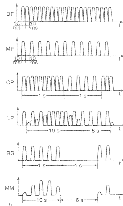
Ryc. 9.6. Elektrody okrągłe małe w uchwycie nieruchomym (a). Rodzaje prądów diadynamicznych (b).
