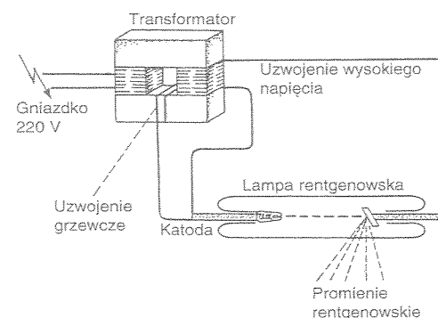
Ryc. 8.1. Schematyczne przedstawienie aparatu rentgenowskiego (wg Son nabenda/Benza).
